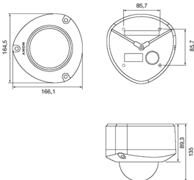
Wymiary kamery
